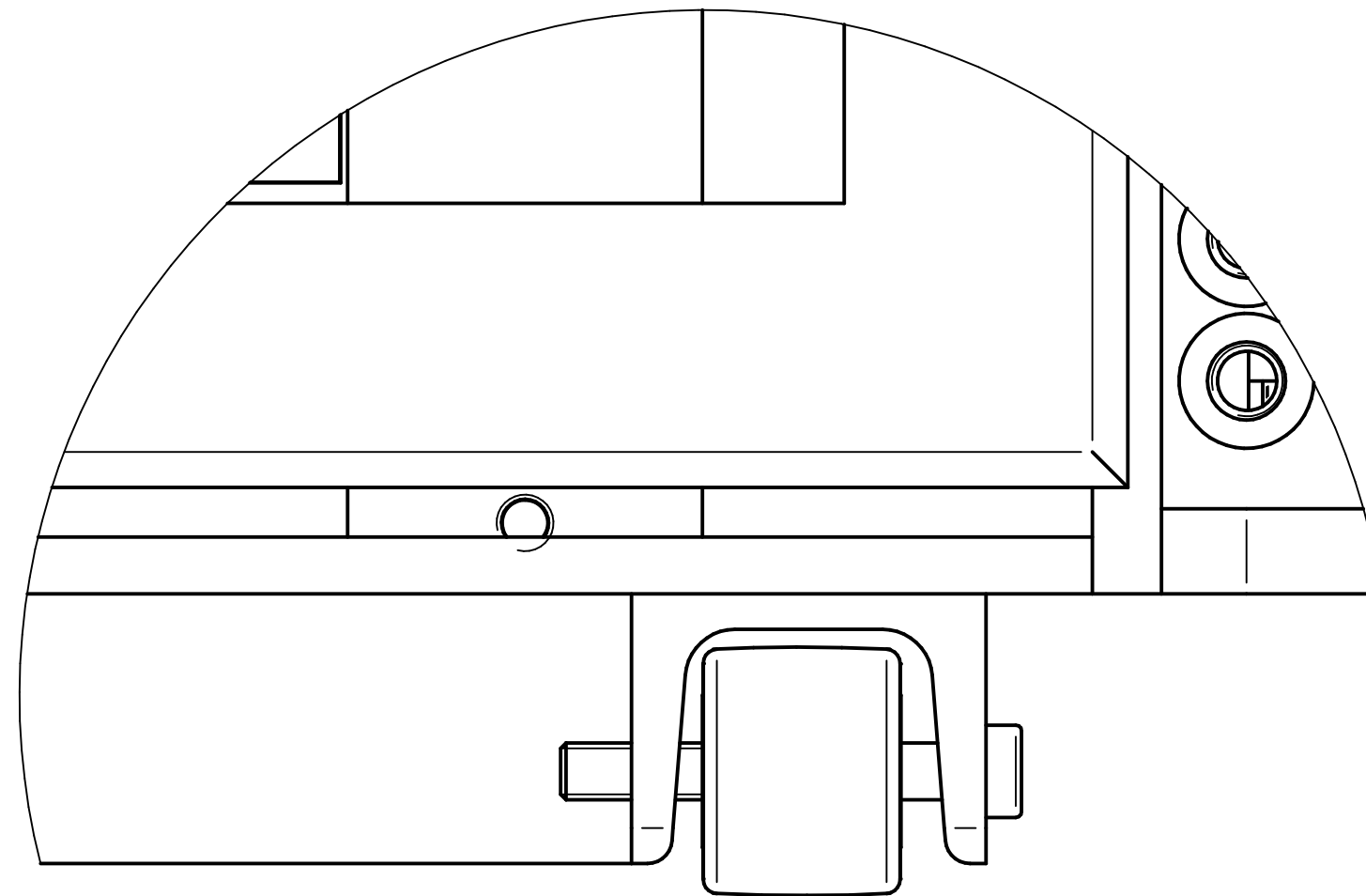
DETAIL A 1:1
