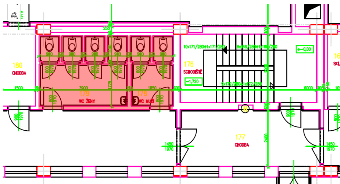
REKONSTRUKCE TOALET STRAVOVACÍHO PROVOZU V 1.NP OBJEKTU O
