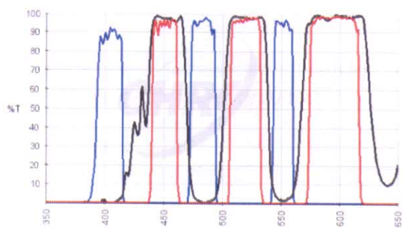
třípásmový filtr B/G/R
