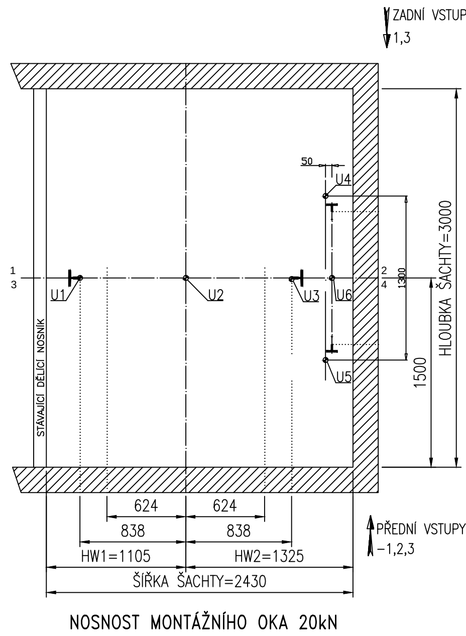
POHLED NA MONTÁŽNÍ OKA VE STROPU ŠACHTY
