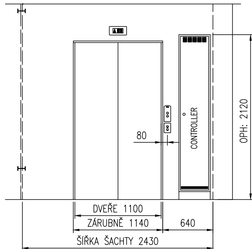
POHLED NA ROZVADĚČ A DVEŘE VE STANICI "3"
