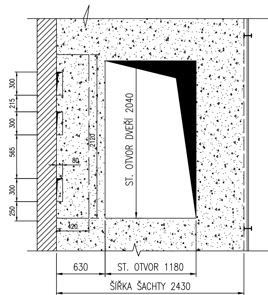
STAVEBNÍ OTVORY PŘI POHLEDU ZE ŠACHTY
